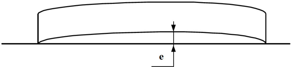
Рис. 9 Отклонение от прямолинейности (кривизна)
